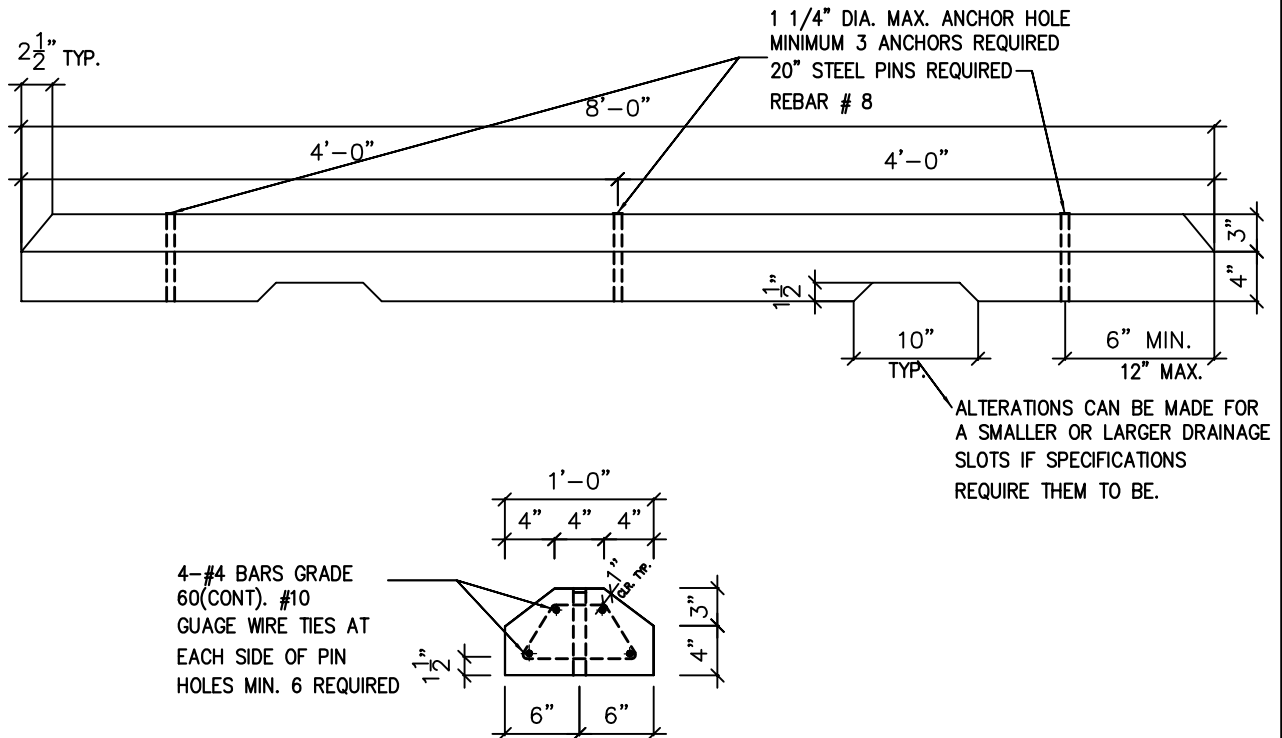
1 8' PRECAST CONCRETE WHELL STOP ST7|ST8 SCALE: N.T.S.
